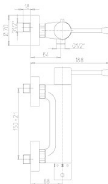
Schéma technique
