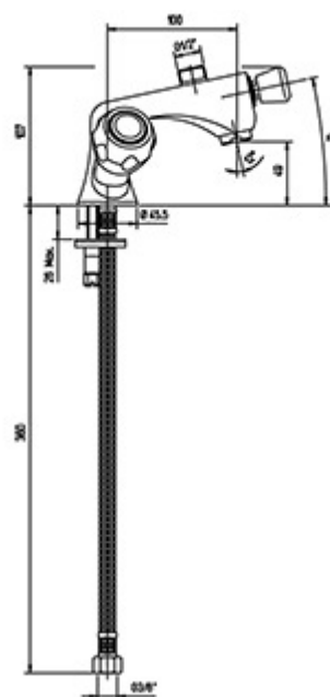
Schéma technique
