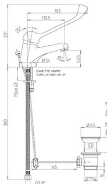
Schéma technique
