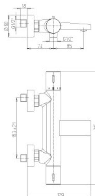
Schéma technique
