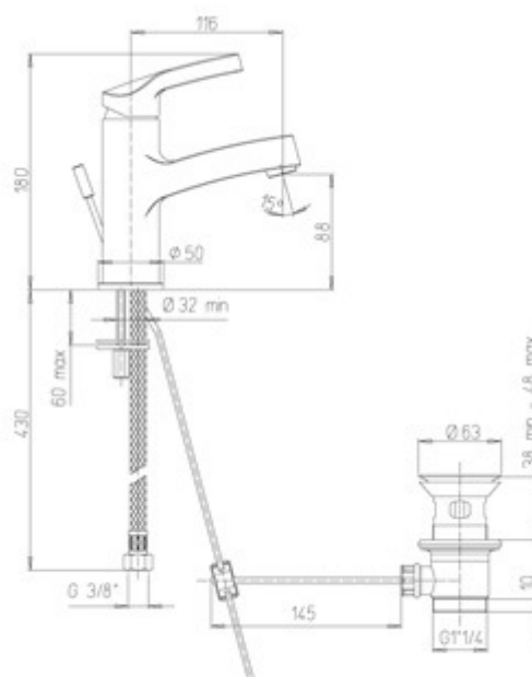
Schéma technique
