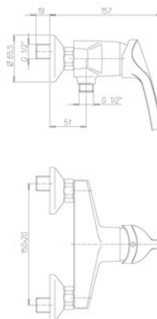
Schéma technique
