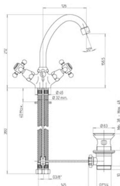
Schéma technique
