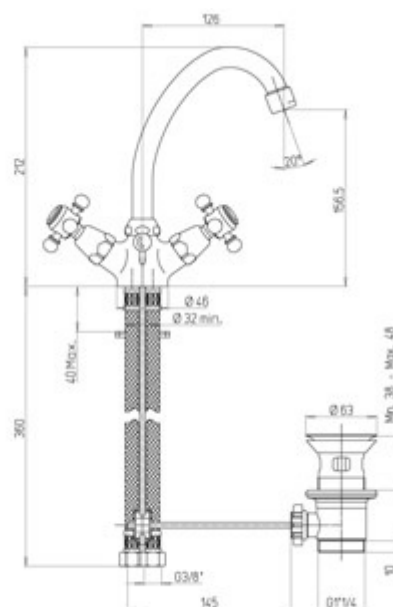
Schéma technique
