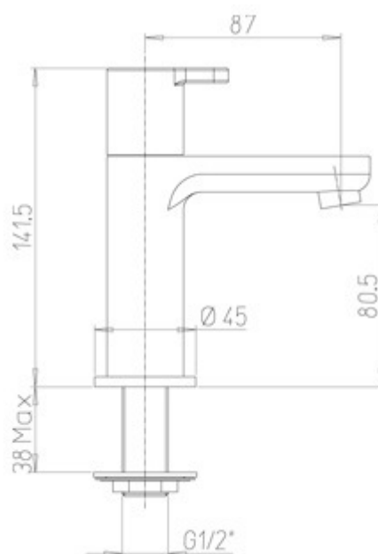
Schéma technique
