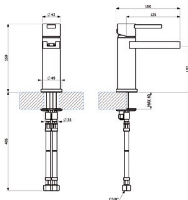
Schéma technique
